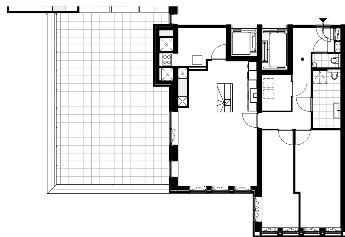
Basis plattegrond 1 : 150
