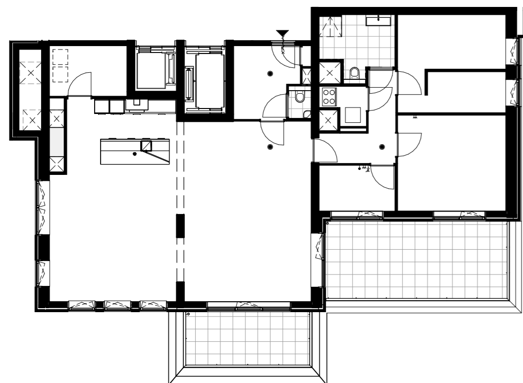
Basis plattegrond 1 : 150
