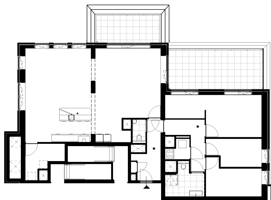
Basis plattegrond 1 : 150
